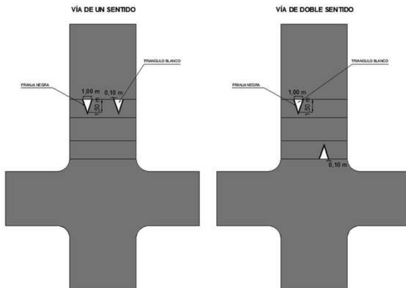
Figura 5 d Demarcación Acera continua
