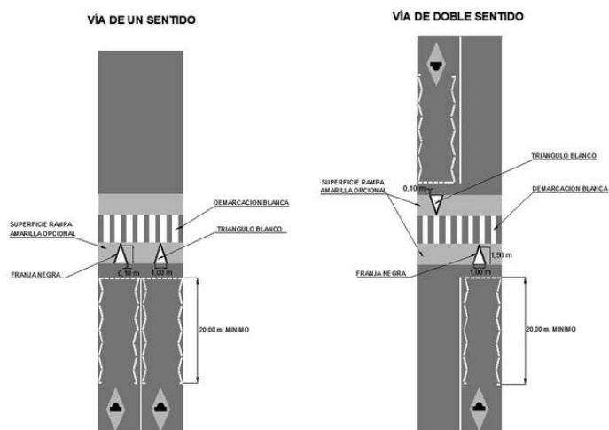
Figura 5 c Demarcación Lomo de toro Plano Vía Urbana
