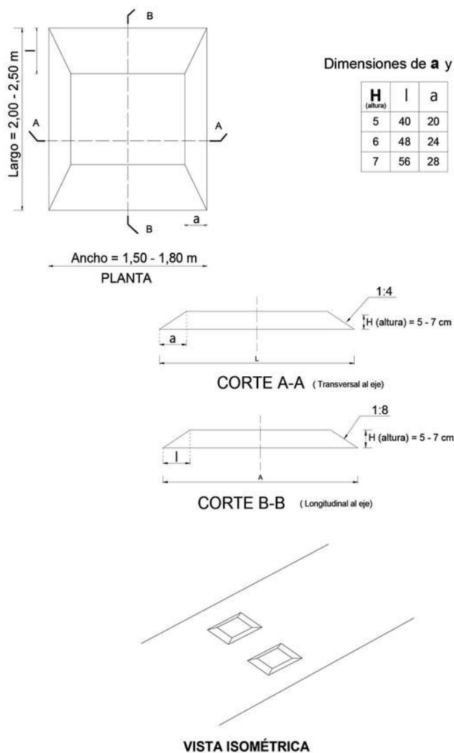
Figura 6 a Diseño geométrico Cojines
