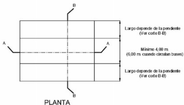
Figura 1b Diseño Geométrico - Lomo de Toro Plano
