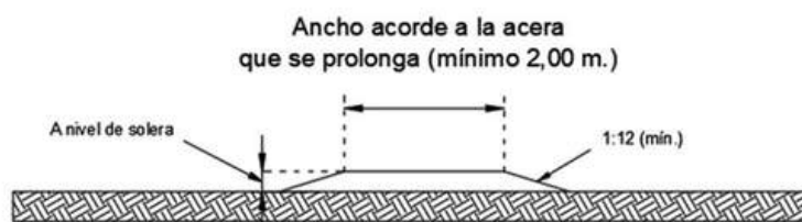
CORTE B-B
