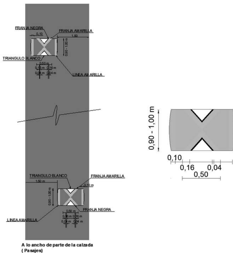
Figura 5 f Demarcación Lomillos en pasajes (excepto aquellos con material retrorreflectante incorporado en su fabricación)
