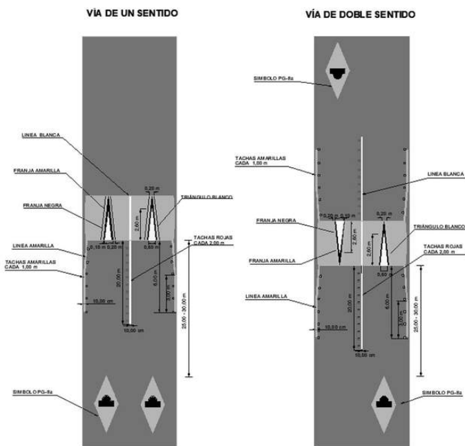
Figura 5 b Demarcación Lomo de toro redondeado Vía Urbana
