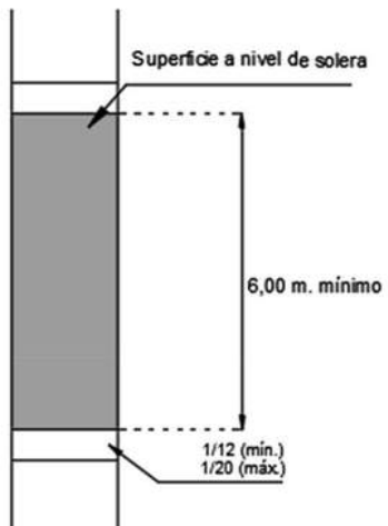
TRAMO PLANTA
