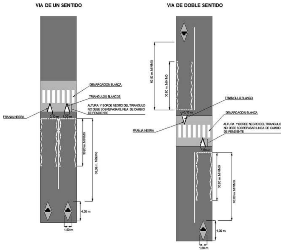
Figura 5 d Demarcación Acera continua
