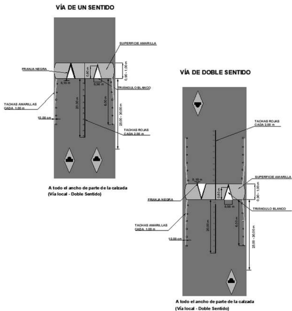
Figura 5 h Demarcación Lomillos en vía local (Excepto aquellos con material retrorreflectante incorporado en su fabricación) Alternativa N° 2
