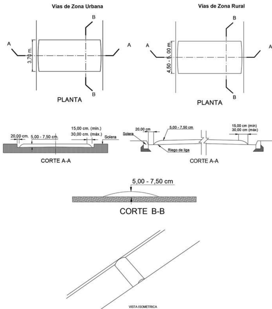
Figura 1a Diseño Geométrico – Lomo de Toro redondeado
