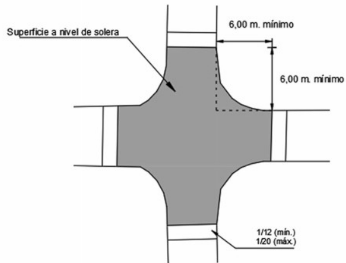
Figura 3a Diseño Geométrico - Plataforma
