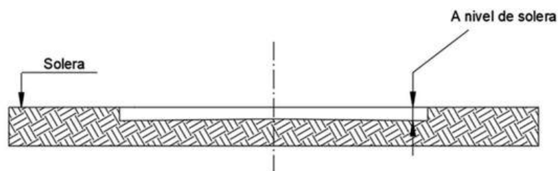
CORTE A-A
