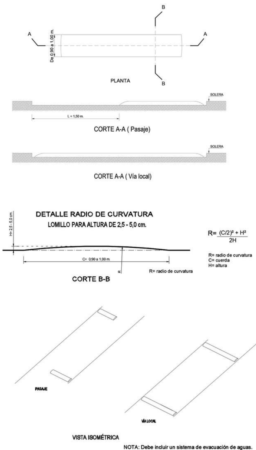
Figura 4 Diseño Geométrico - Lomillo
