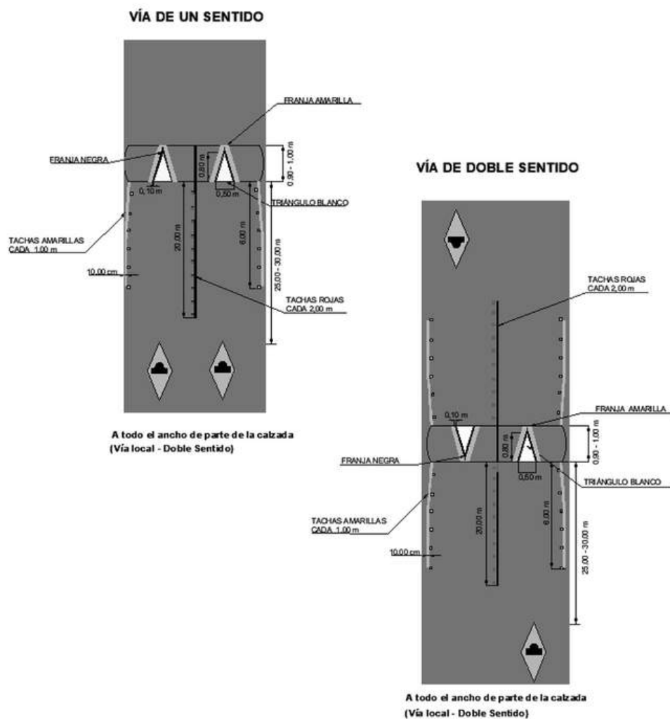
Figura 5 g Demarcación Lomillos en vía local (Excepto aquellos con material retrorreflectante incorporado en su fabricación) Alternativa N° 1
