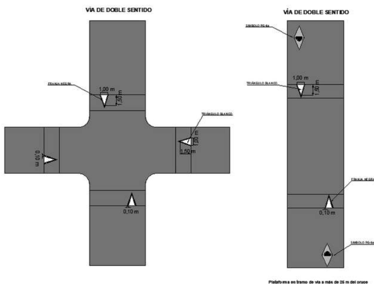
Figura 5 f Demarcación Lomillos en pasajes (excepto aquellos con material retrorreflectante incorporado en su fabricación)
