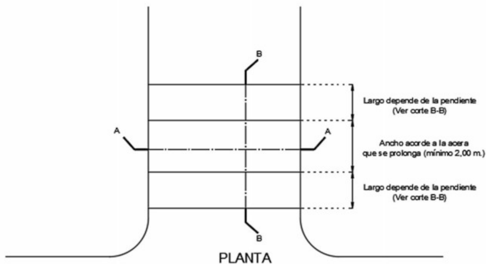
Figura 2 Diseño Geométrico - Acera Continua
